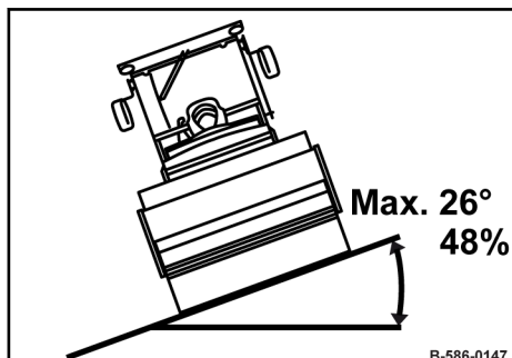
Fig. 11: Máxima inclinación transversal
