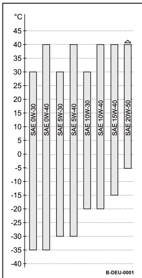
Fig. 156: Diagrama de viscosidad de aceites
